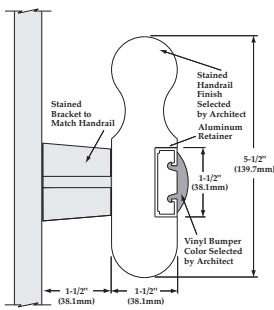
HW20
