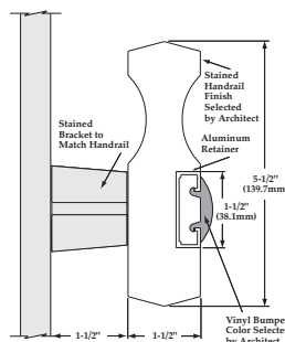
HW40
