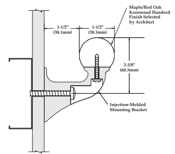
HW70
