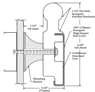
HW60
